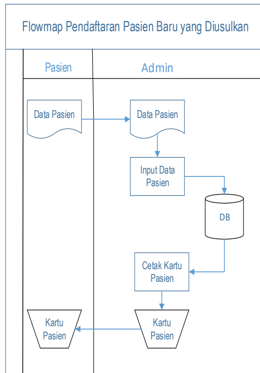
Gambar 3. Flowmap Pendaftaran Pasien baru yang di usulkan
